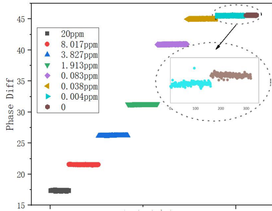
Figure 2 测量范围广，兼顾高低溶解氧浓度测量
